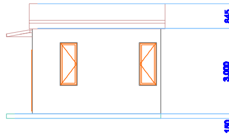
RIGHT ELEVATION
